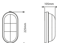
Светильник "Изумруд-2"
