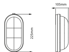
Светильник "Изумруд-3"
